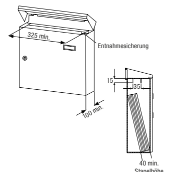
senkrechte Kästen Form A Einwurf oben
